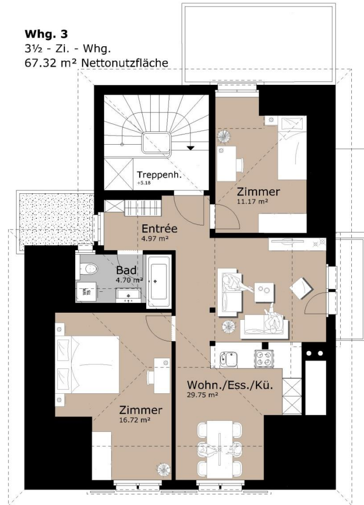
Dachgeschoss
