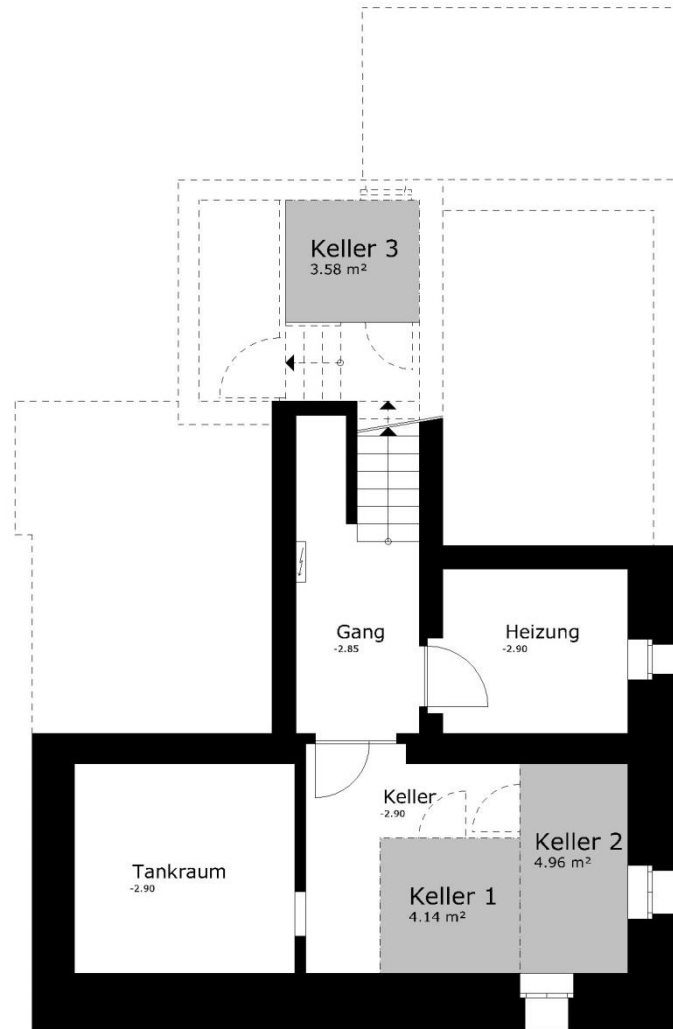
Untergeschoss
