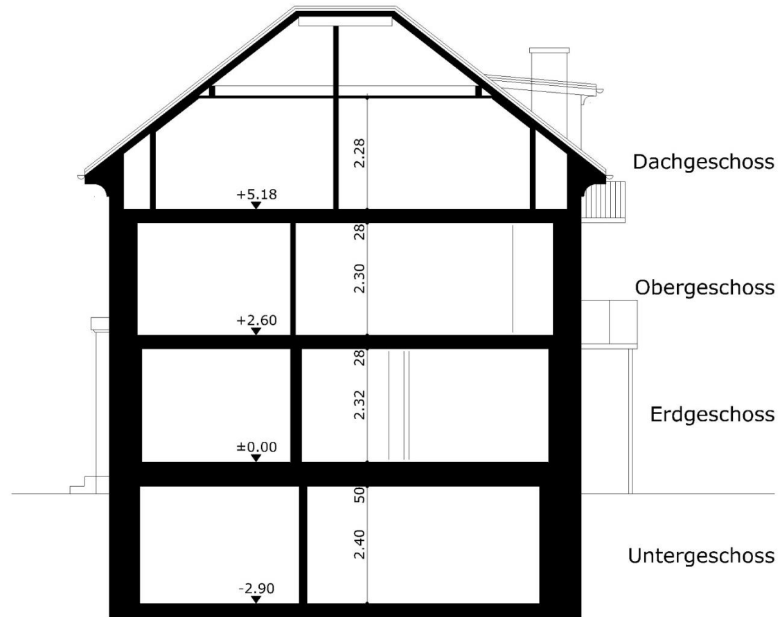
Schnitt
